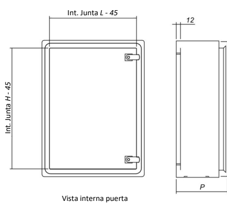
Vista interna puerta
