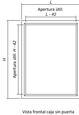
Vista frontal caja sin puerta
