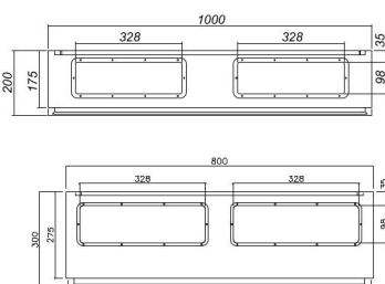
Vista interna puerta izquierda
