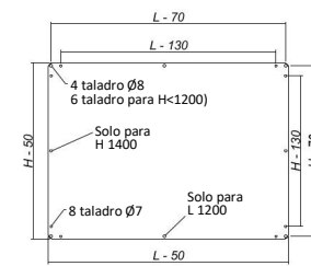
Vista placa de montaje
