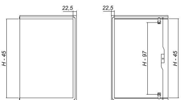
Vista interna puerta izquierda
