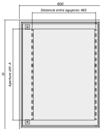
Vista frontal caja con bastidor rack 19"
