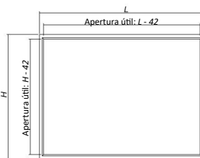
Vista frontal caja sin puerta
