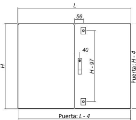
Vista frontal caja con puerta
