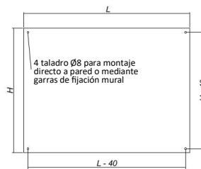
Vista posterior caja
