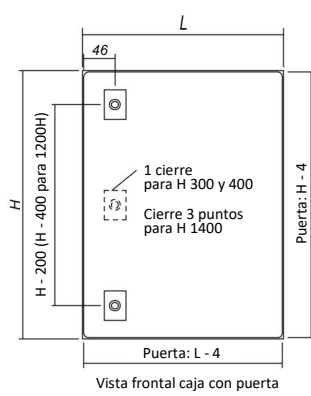
Vista frontal caja con puerta
